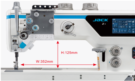
超大空间：放料轻松转角无忧，大容量梭芯
