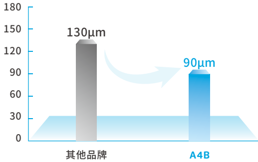
振动降低23% (降至90μm)
