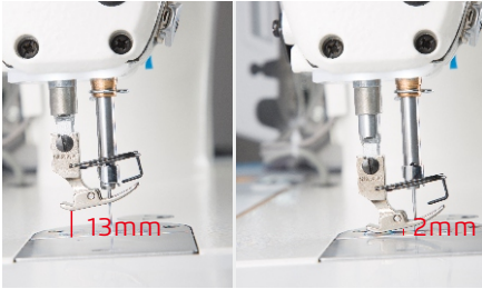
步进控制，高度可调
